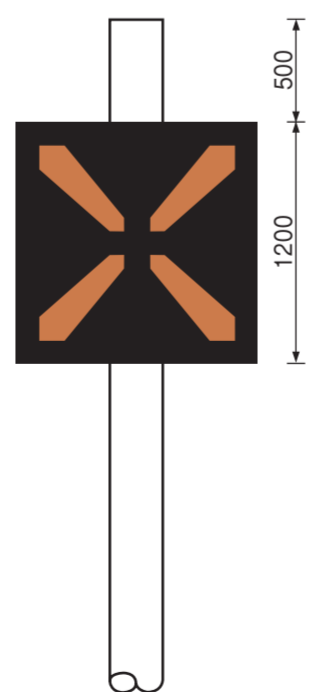
【信号柱の標識】
